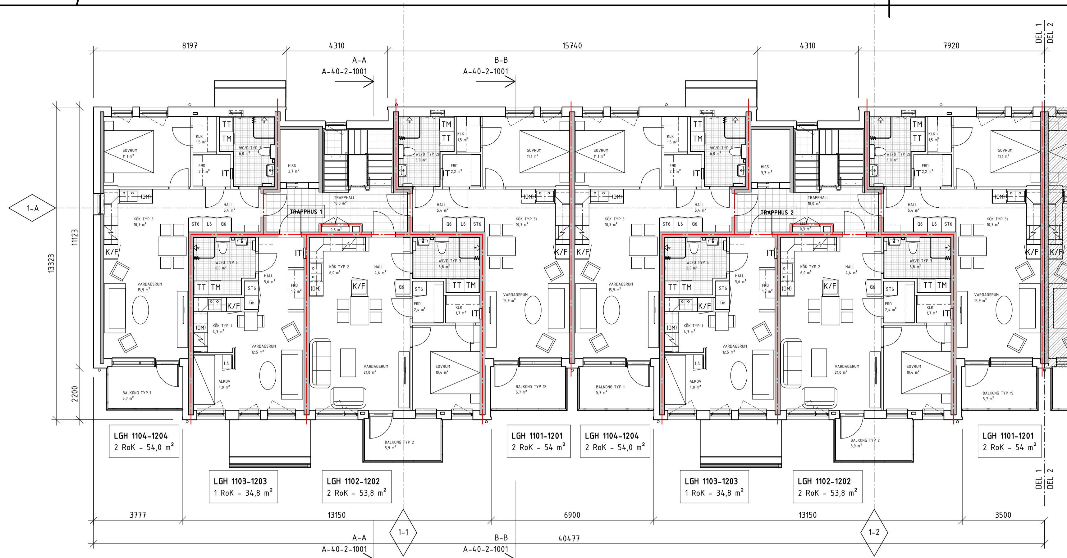
PLAN 11-12 - DEL 1
