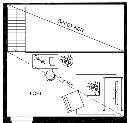
UTRYMNINGSDÖRR
