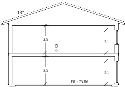
SEKTION A-A
