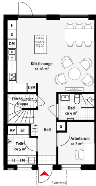
Alt. 3 Kök med köksö + arbetsrum
