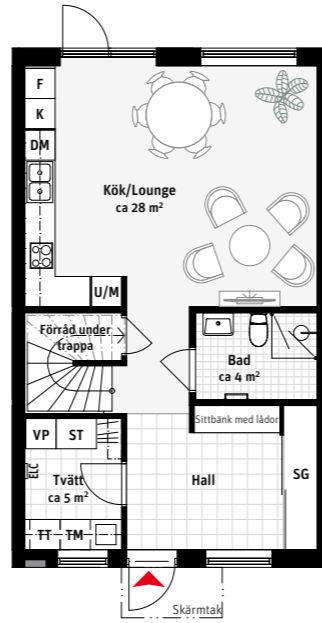
Alt. 2 Kök + inredd hall
