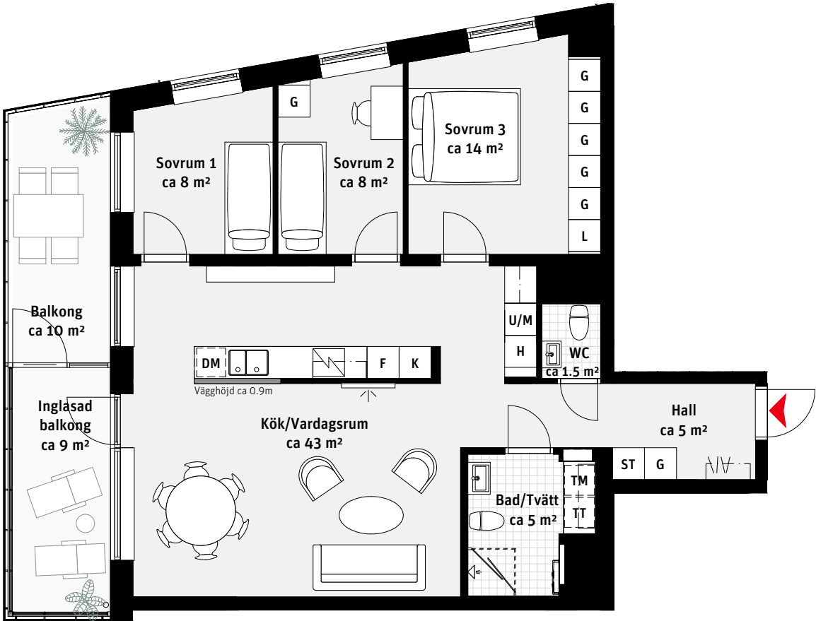
Grundutförande
