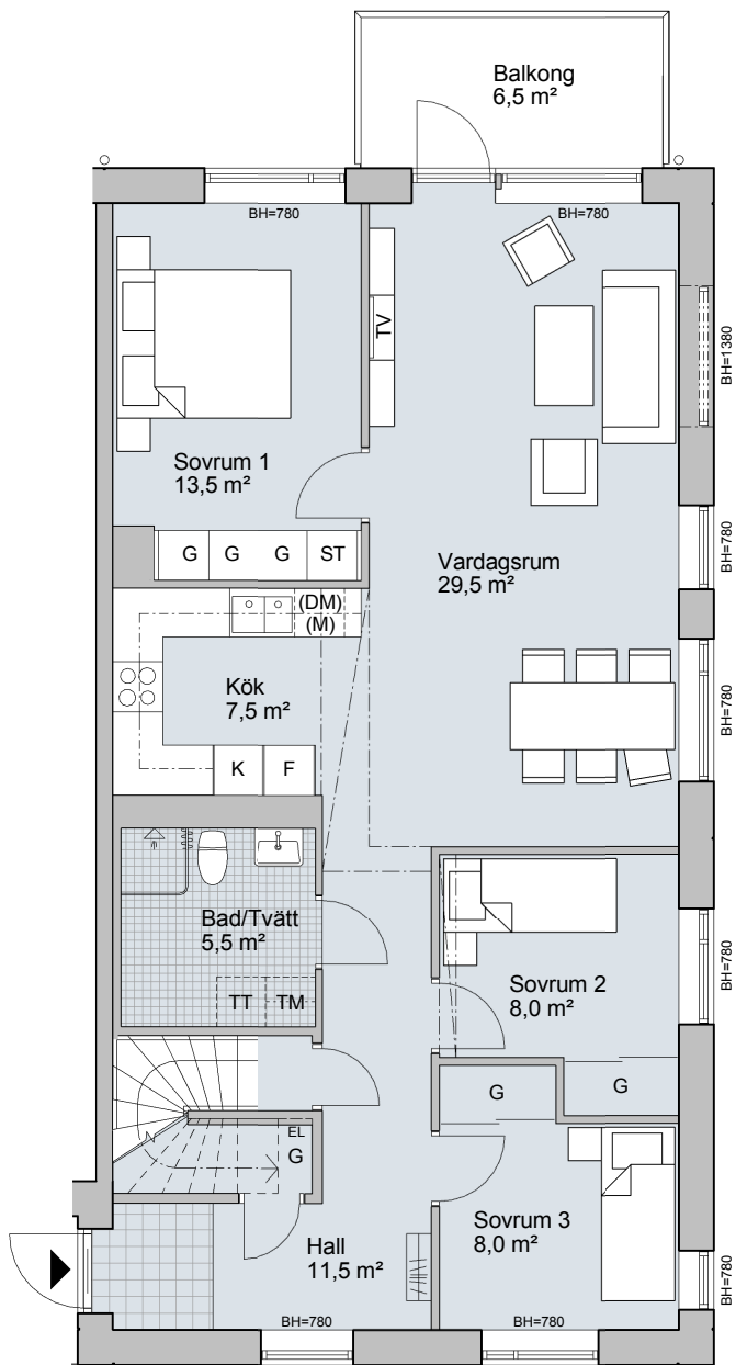
Våning 4
